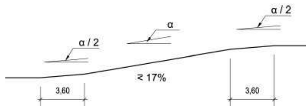
2. ábra: az álláshelyekhez vezető lejtő (közlekedési rámpa)
